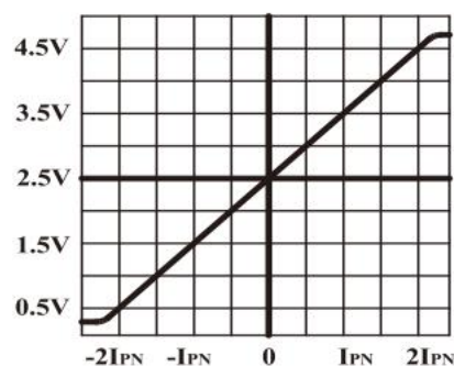
输入电流—输出电压
